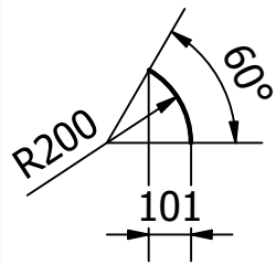
CHI TIẾT 1: Vỏ mái - số lượng 1 - TL: 1:20
