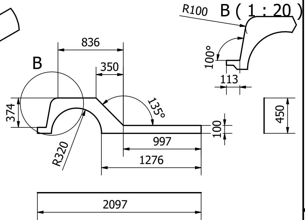
CHI TIẾT 3: Vỏ bánh sau - SL 2 - TL 1:30
